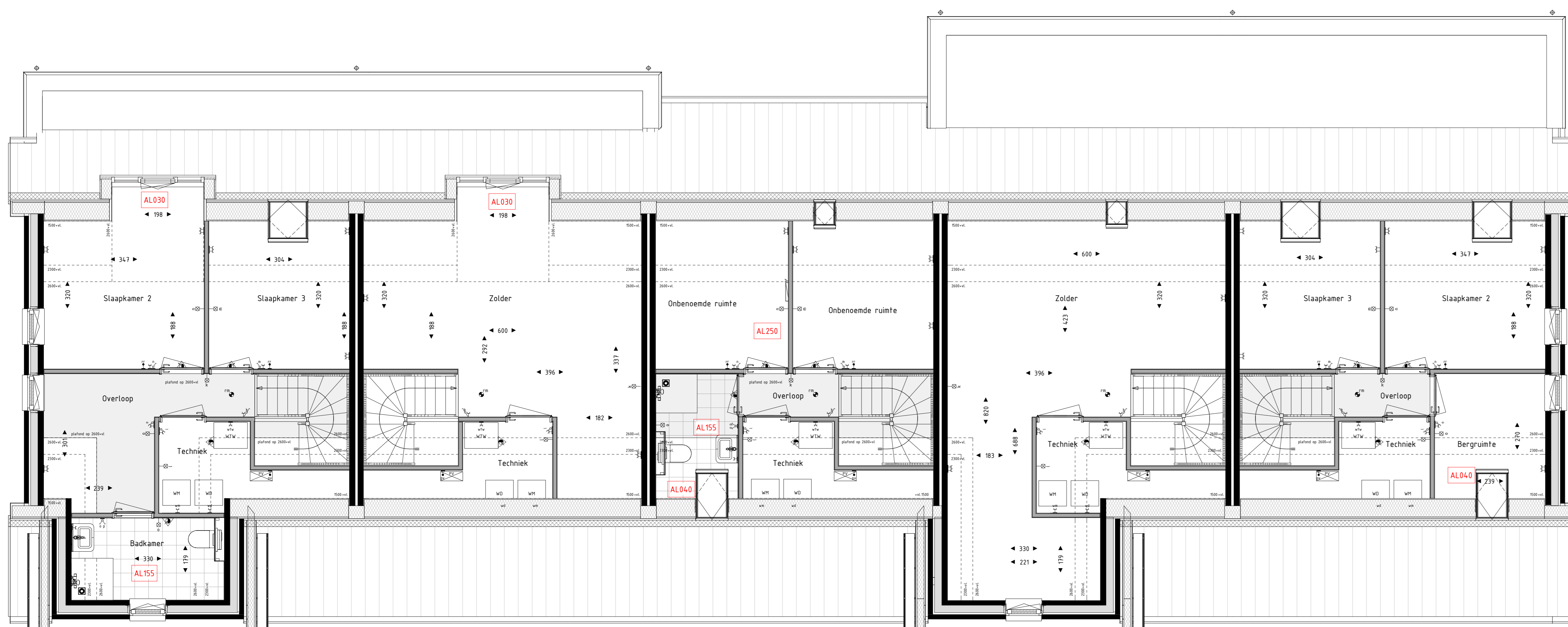
Eerste verdieping
