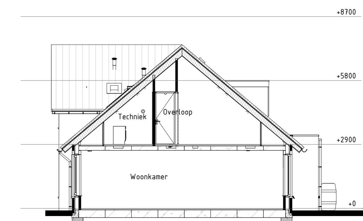
Dwarsdoorsnede
