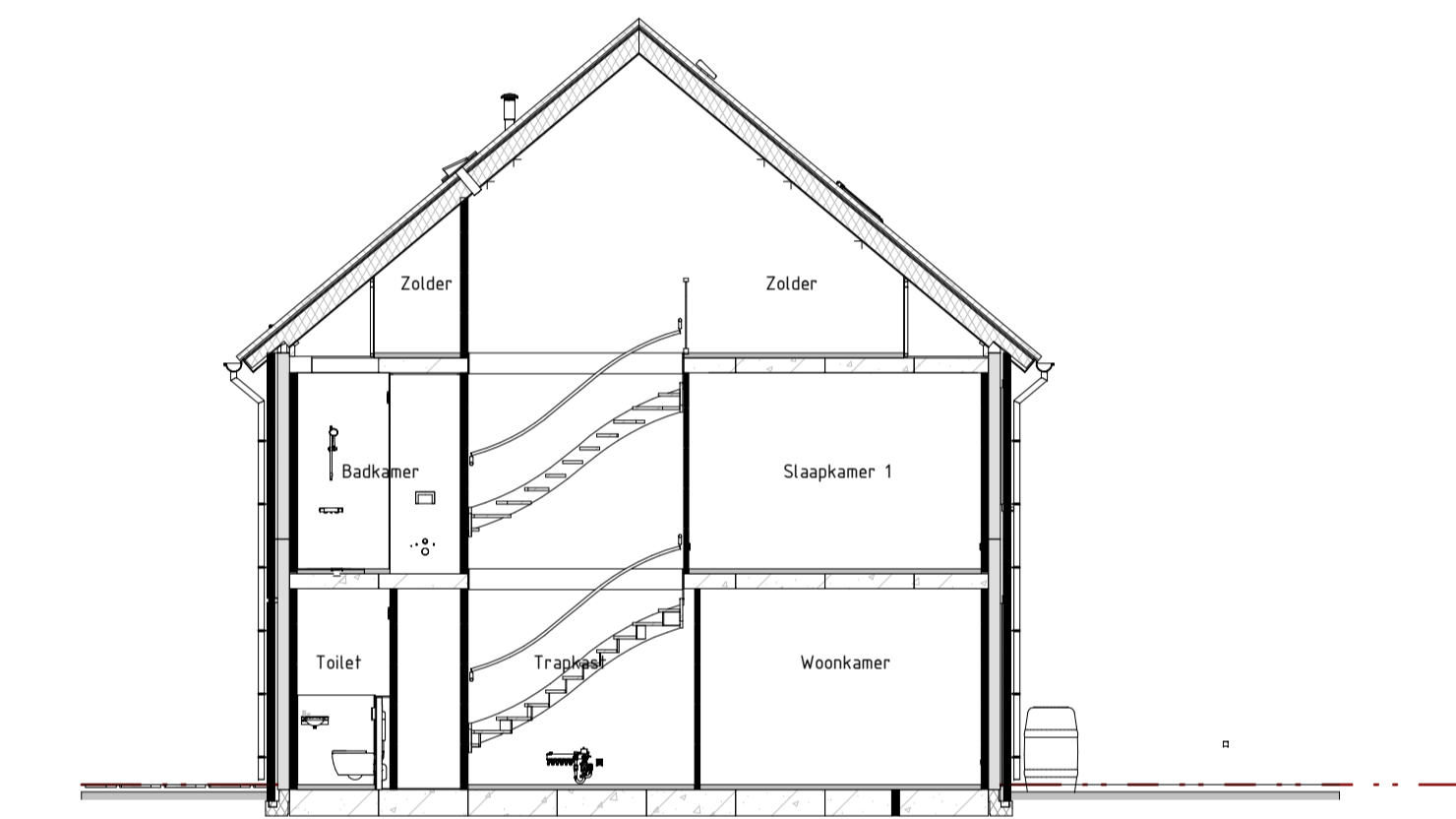
Dwarsdoorsnede
