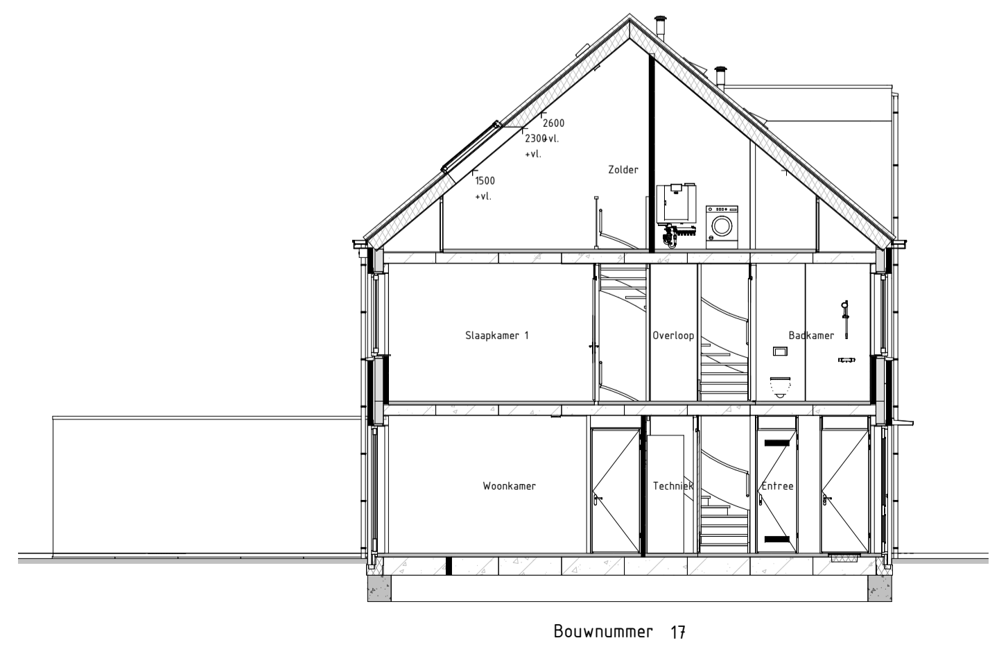
Doorsnede AA
